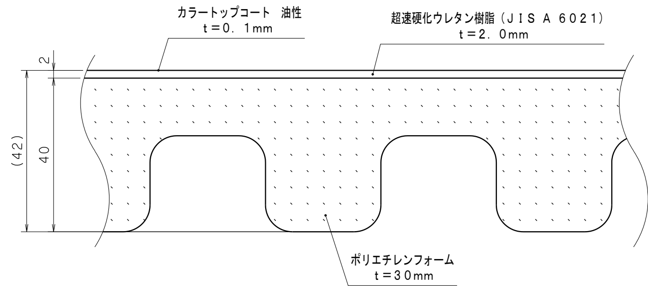
断面図 S = 1 / 1
