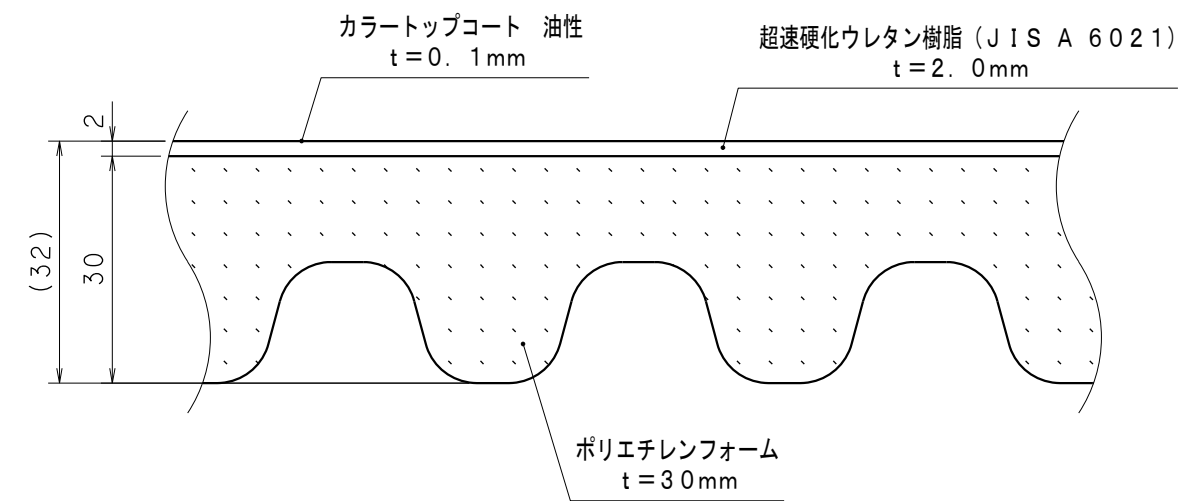
断面図 S = 1 / 1
