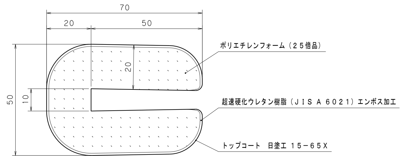
詳細図 S = 1 / 1
