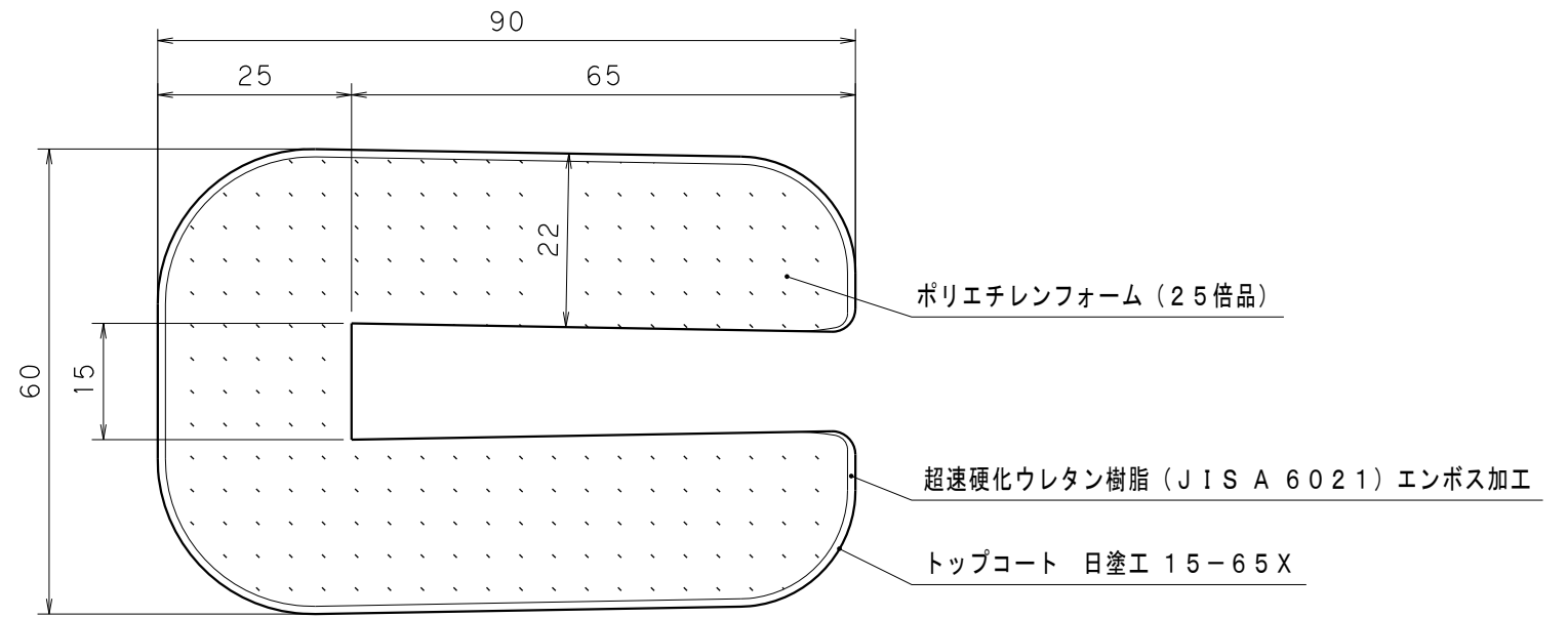
詳細図 S = 1 / 1
