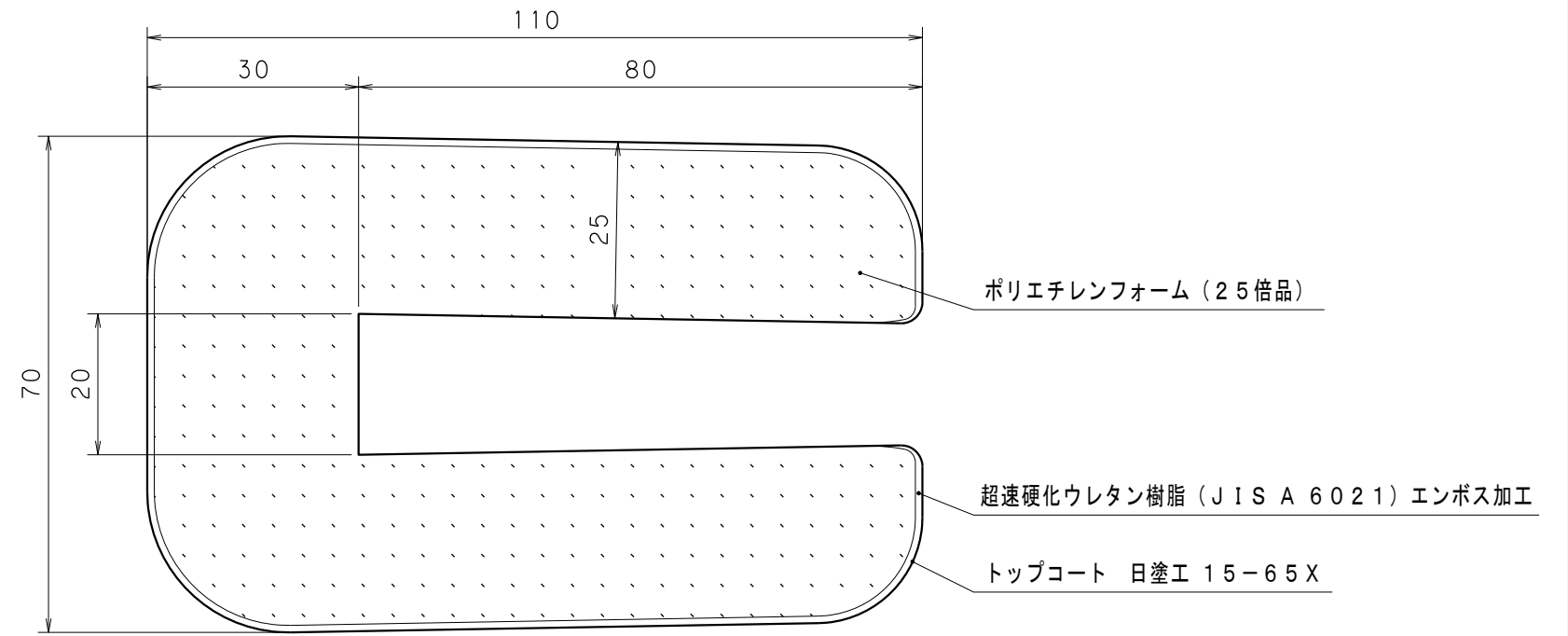
詳細図 S = 1 / 1
