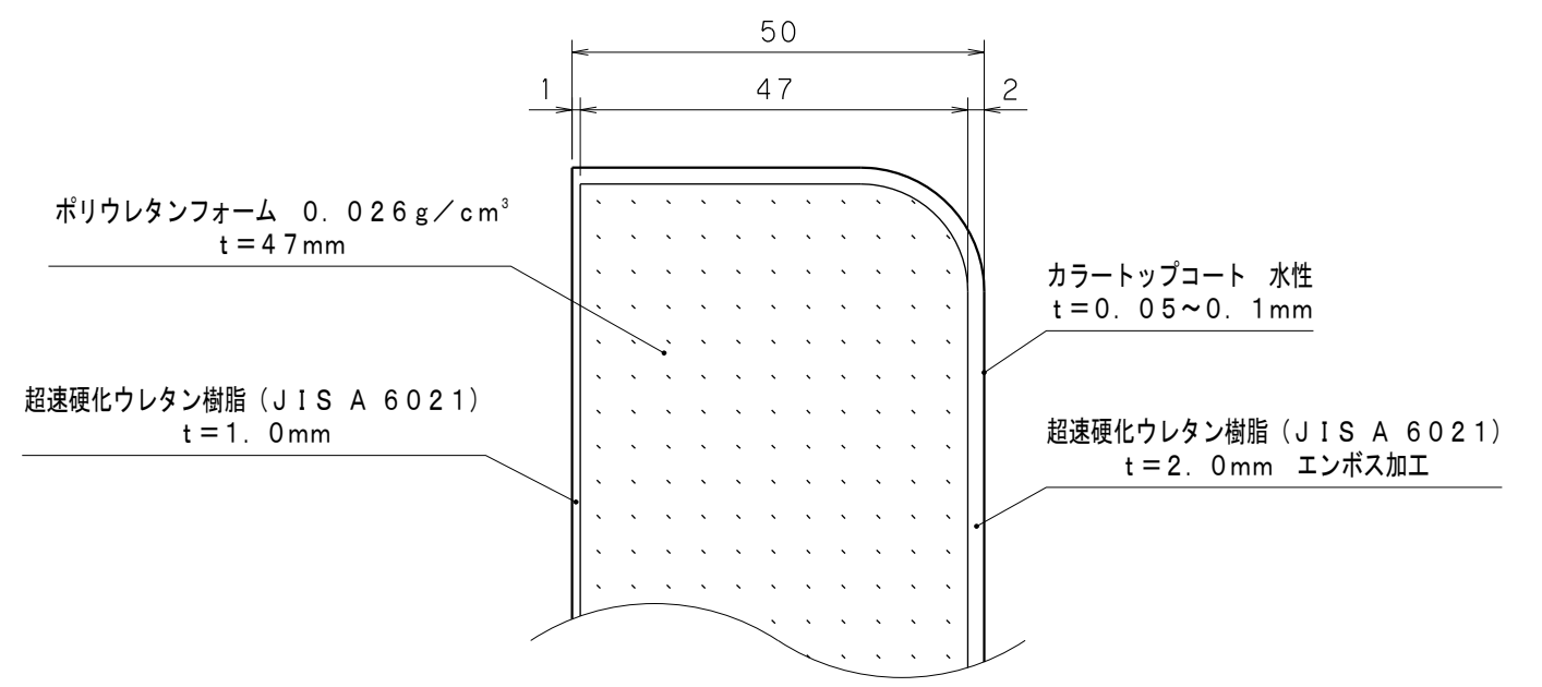
断面図 S = 1 / 1
