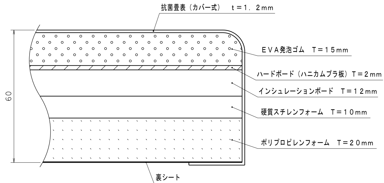
断面図 S=1/1
