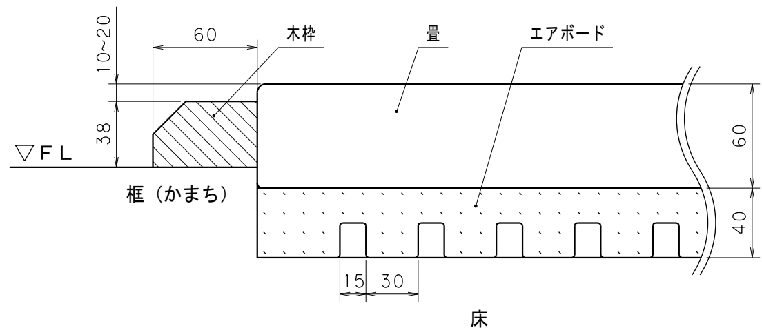
納まり断面図 S = 1 / 3
