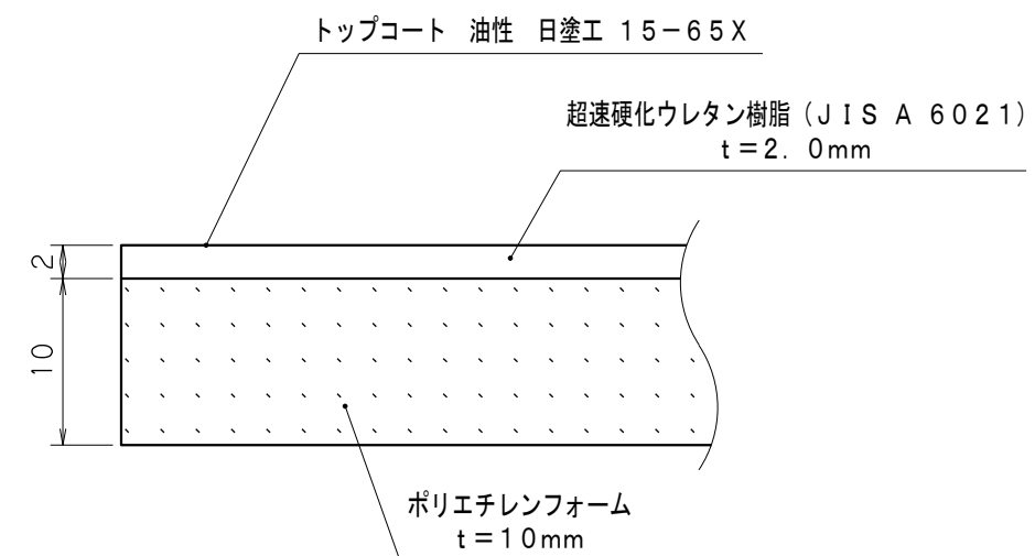
断面図 S = 2 / 1
